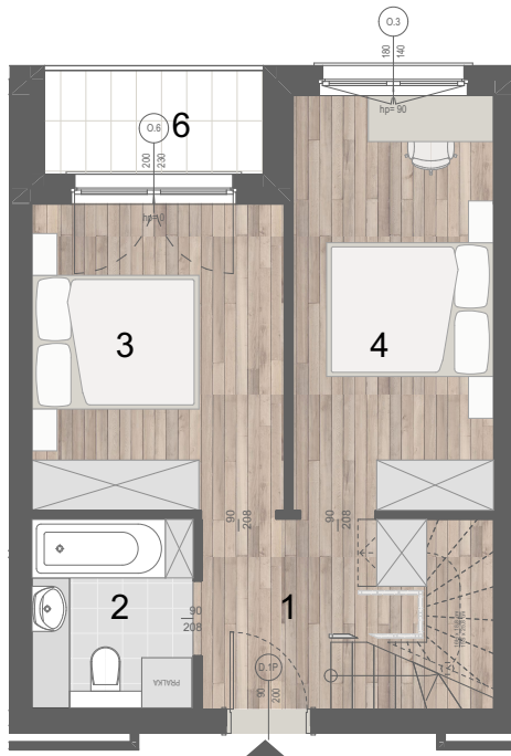
POZIOM 0 MIESZKANIA
